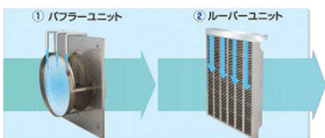
湿式集塵機構部
